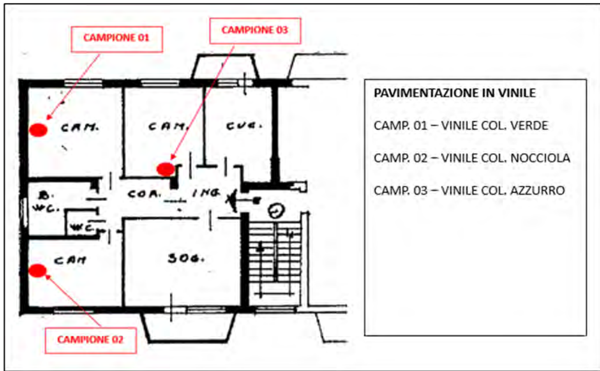
Fig. 1.3.2 – Pianta piano primo, con indicazione punto di prelievo campioni n. 01-02-03
